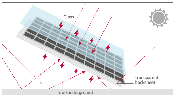
Bifacial module
